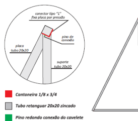
VISÃO LATERAL DO CAVALETE - 50 x 100 cm
