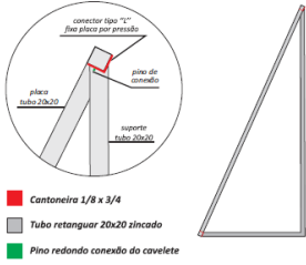
VISÃO LATERAL DO CAVALETE - 50 x 110 cm
